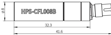
图 3. HPS-CFL008B 传感头
