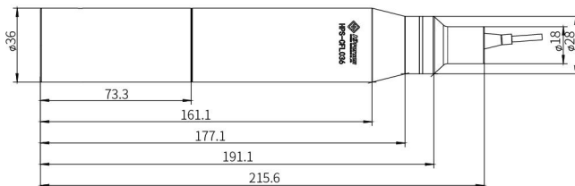
图 9. HPS-CFL036 传感头
