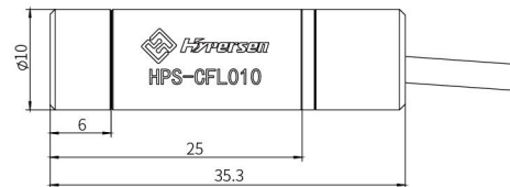
图 4. HPS-CFL010 传感头
