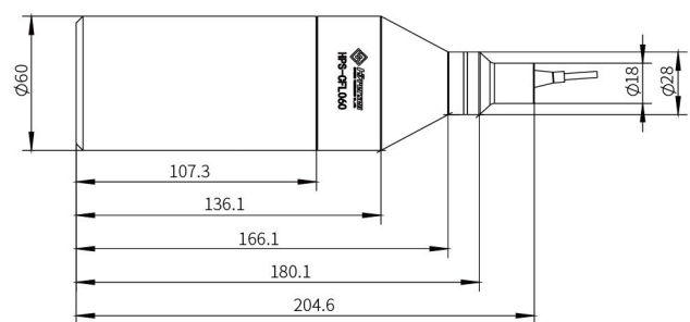
图 18. HPS-CFL060传感器头
