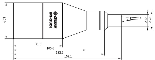
图 16. HPS-CFL053传感器头
