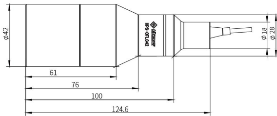
图 13. HPS-CFL042传感器头
