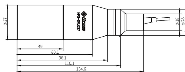
图 10. HPS-CFL037 传感头
