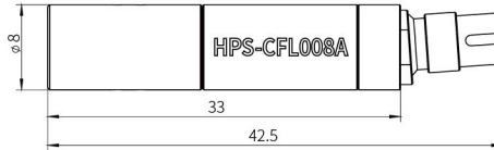
图 2. HPS-CFL008A 传感头
