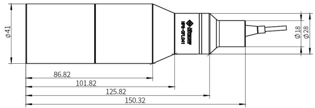
图 12. HPS-CFL041传感器头
