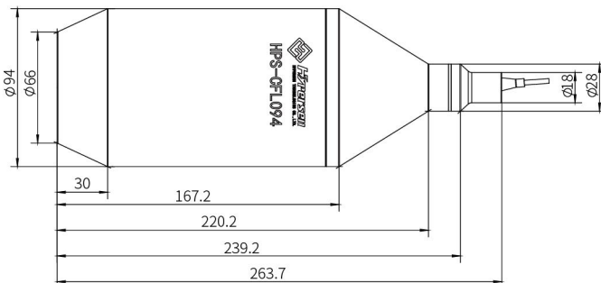
图 19. HPS-CFL094传感器头
