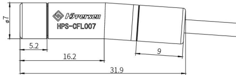
图 1. HPS-CFL007传感头
