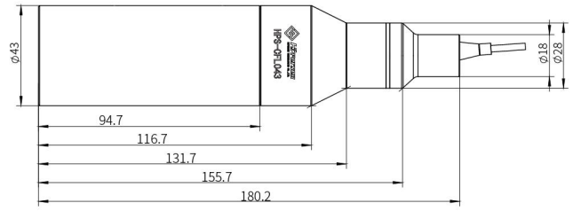
图 14. HPS-CFL043传感器头
