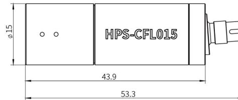
图 6. HPS-CFL015 传感头
