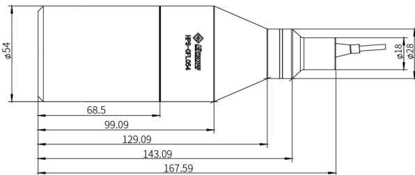
图 17. HPS-CFL054传感器头
