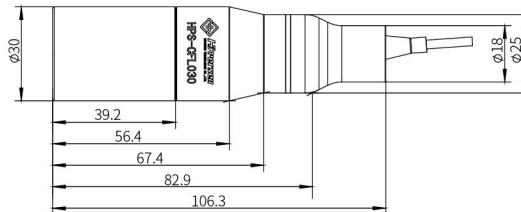
图 8. HPS-CFL030 传感头
