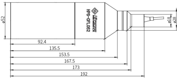
图 15. HPS-CFL052传感器头
