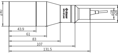
图 11. HPS-CFL040传感器头
