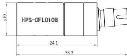
图 5. HPS-CFL010B 传感头
