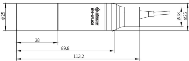
图 7. HPS-CFL025 传感头
